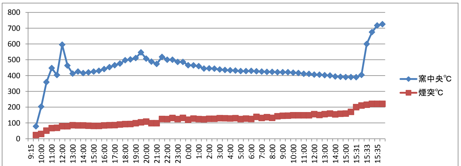
本窯の温度推移
